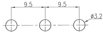
取付穴参考図
