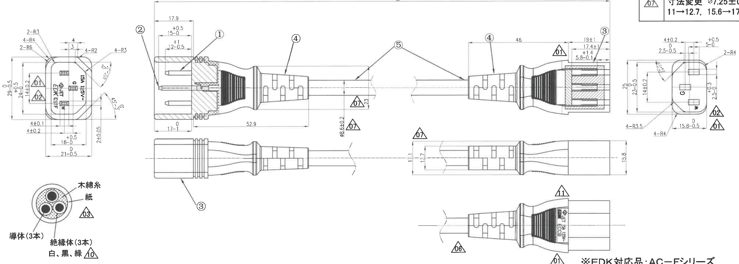
電線断面図 比率 4:1
