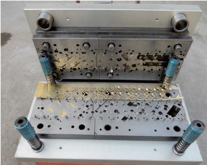
順送プレス金型
