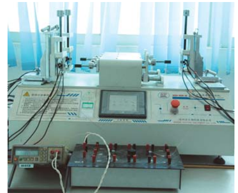
スイッチ / インレット・アウトレット 寿命試験機
