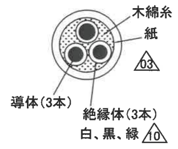
電線断面図 比率 4:1
