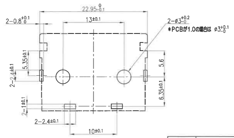
基板取付穴参考図
