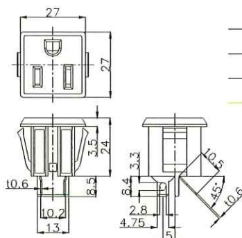
端子参考図
