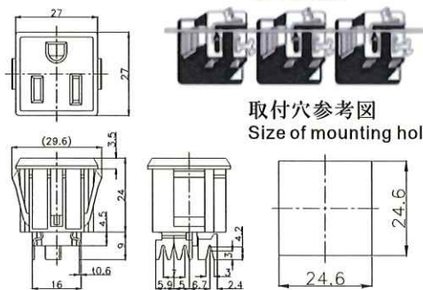
端子参考図
