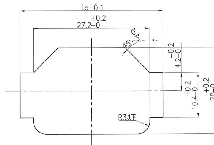
シャーシ取付穴参考図
