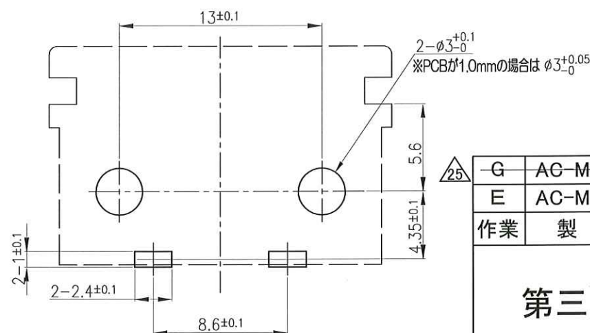
基板取付穴参考図
