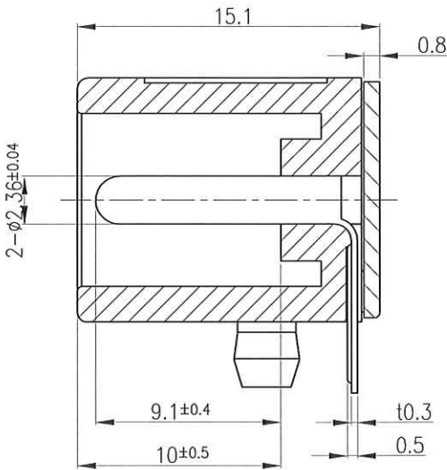
A-A' 断面
