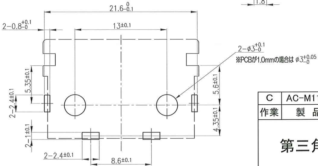
基板取付穴参考図
