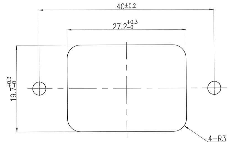
取り付け穴参考図
