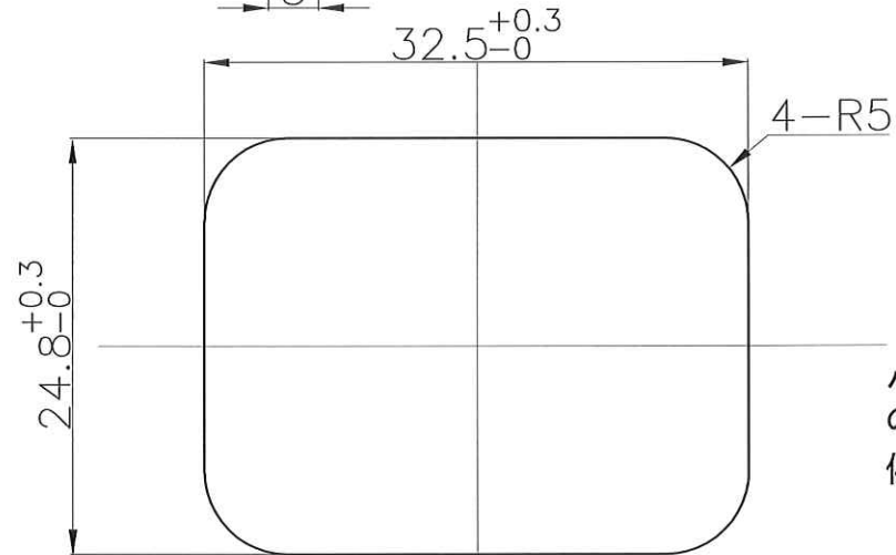
パネル取付穴参考図
