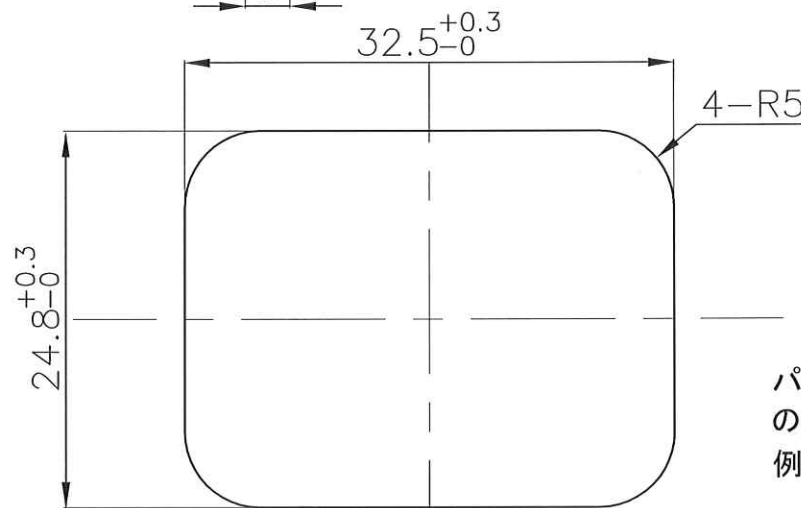
パネル取付穴参考図
