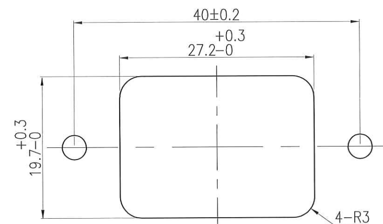
取付穴参考図
