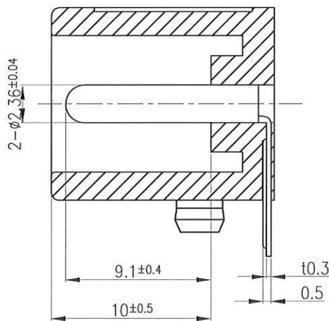
A-A'断面
