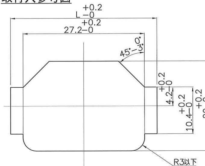
取付穴参考図
