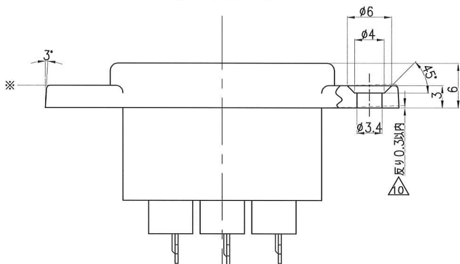
△取付穴参考寸法
