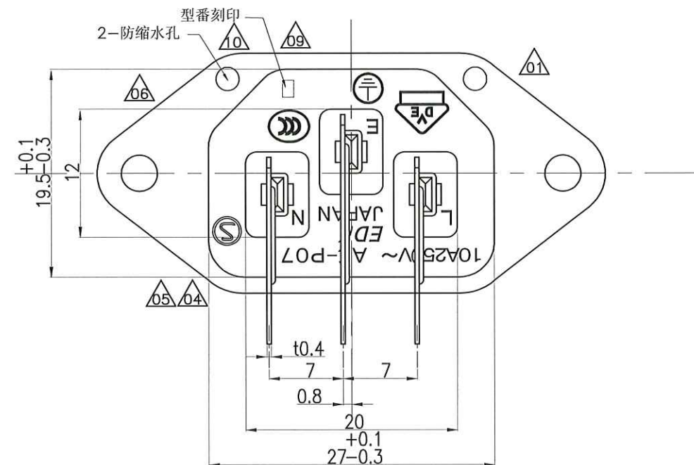
取付穴参考図
