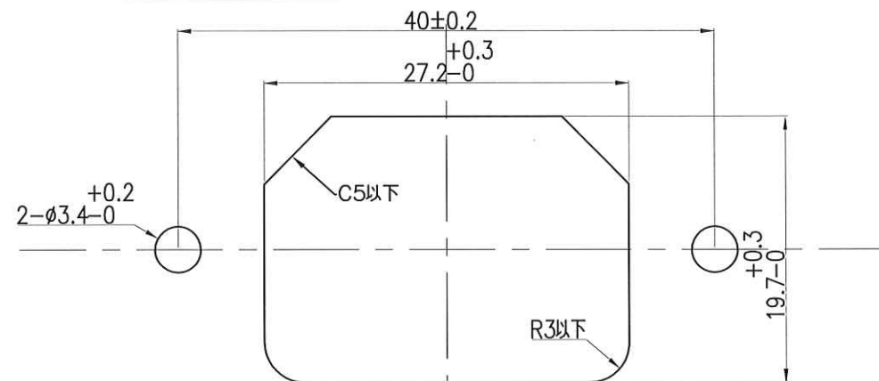
取付穴参考図
