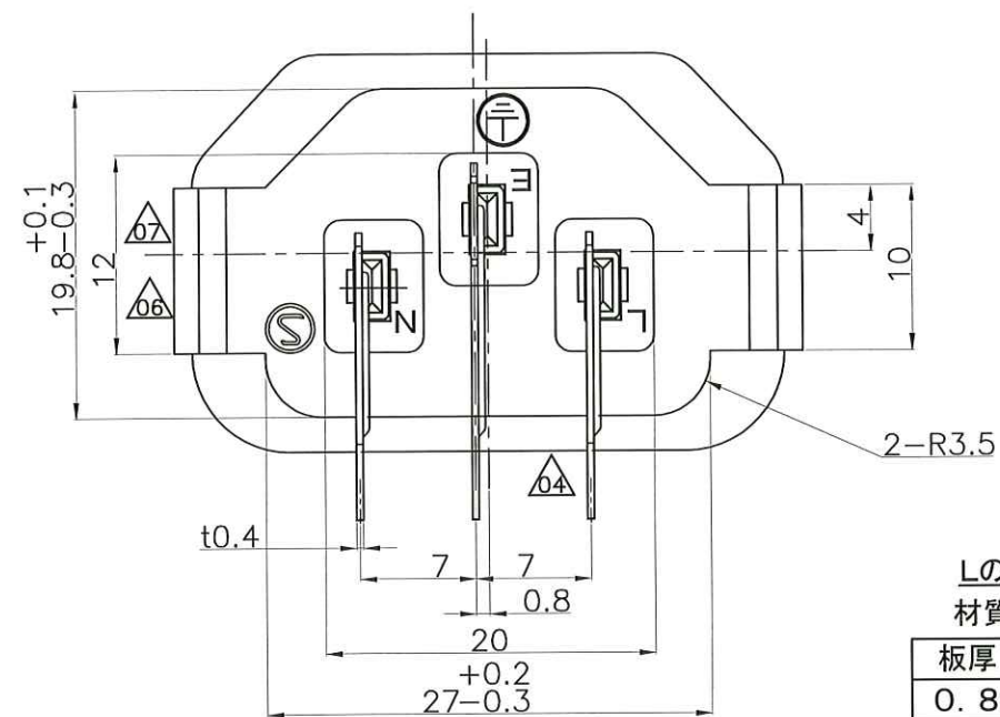
取付穴参考図
