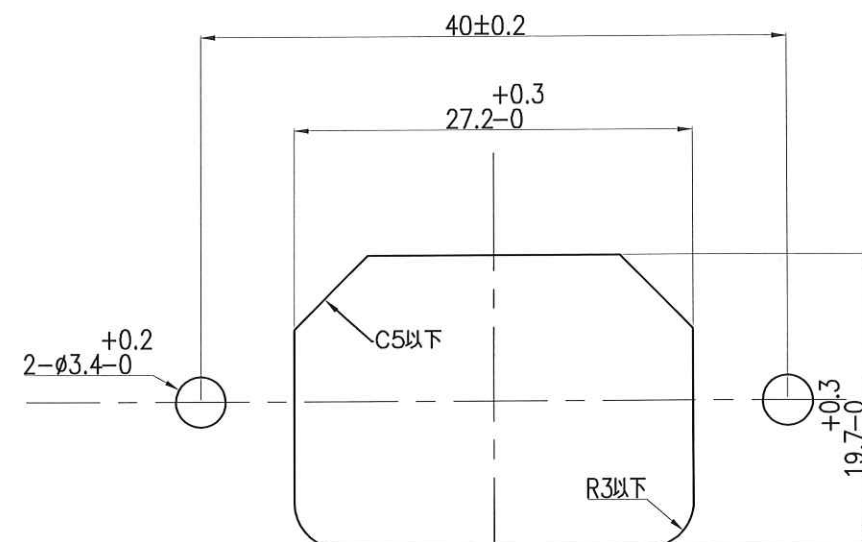
取付穴参考図
