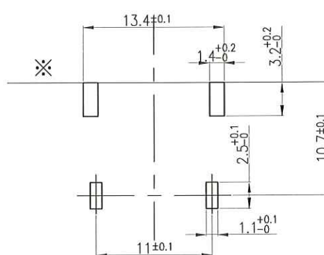
基板取付穴参考図
