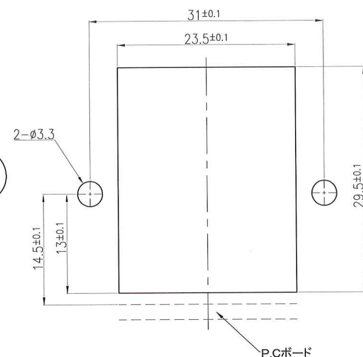
パネル取付穴参考図(2/1)
