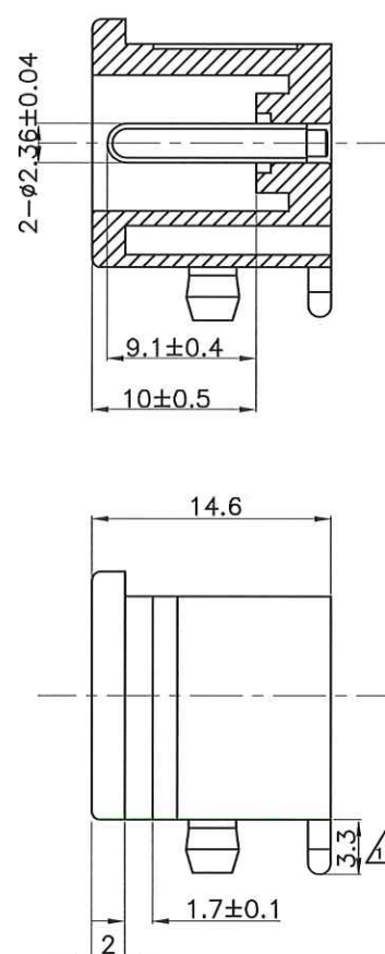
A—A' 断面
