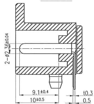
A-A' 断面
