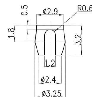
B部詳細図 4/1 (公差±0.1)
