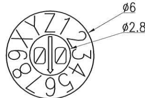
C部詳細図 4/1
