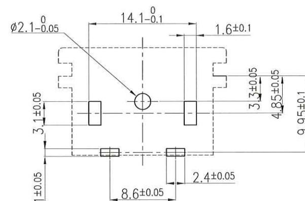
基板穴参考図
