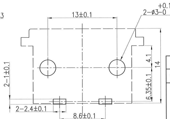
基板取付穴参考図
