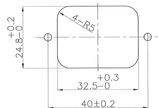
パネル取り付け穴参考図
