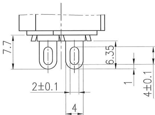
端子形状:A 02
