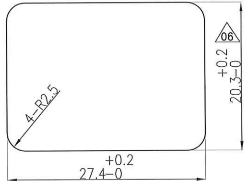
取付穴寸法
